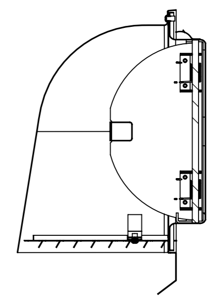
断面図 A-A スケール 1 : 3
