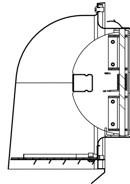
断面図 A-A
