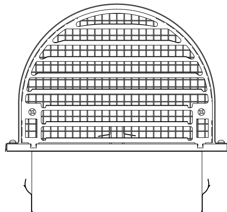
正面図
