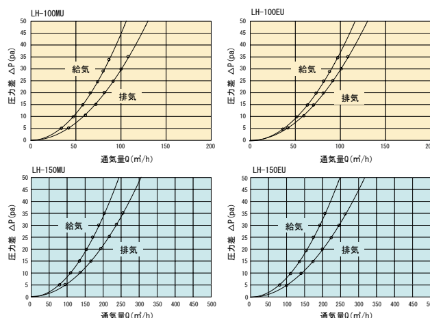
通気量曲線
