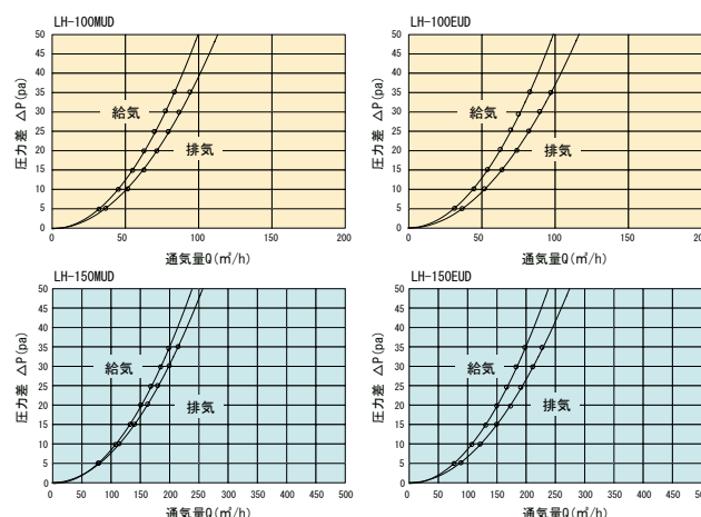
通気量曲線
