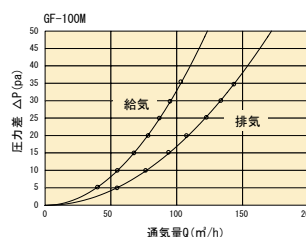
通気量曲線
