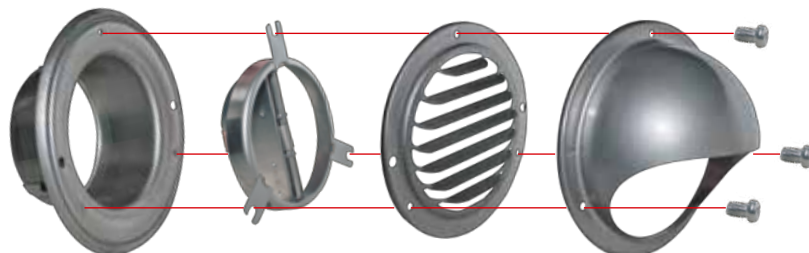
【メンテナンス例】防火ダンパー付きシリーズ：GF100 D
